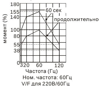
Асинхронный двигатель
